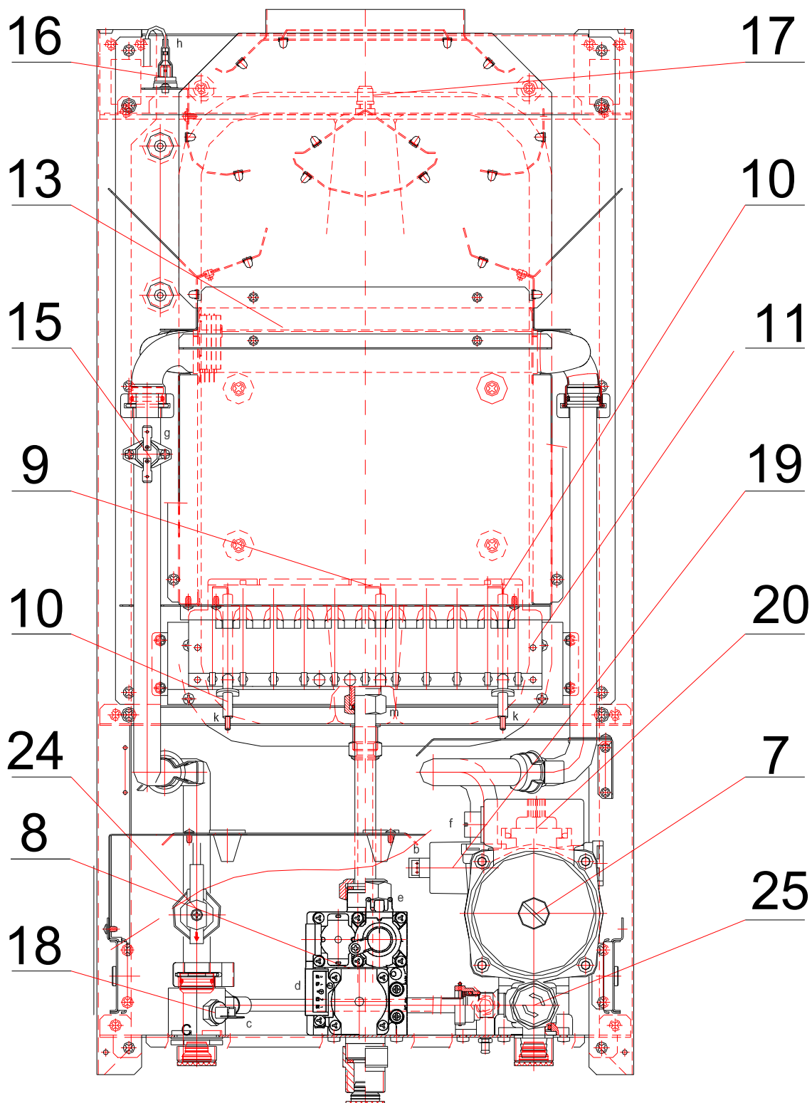
Podstawowe elementy kotła typ Main component of the boiler type Основные элементы котлов типа GCO-13-00, GCO-24-00
