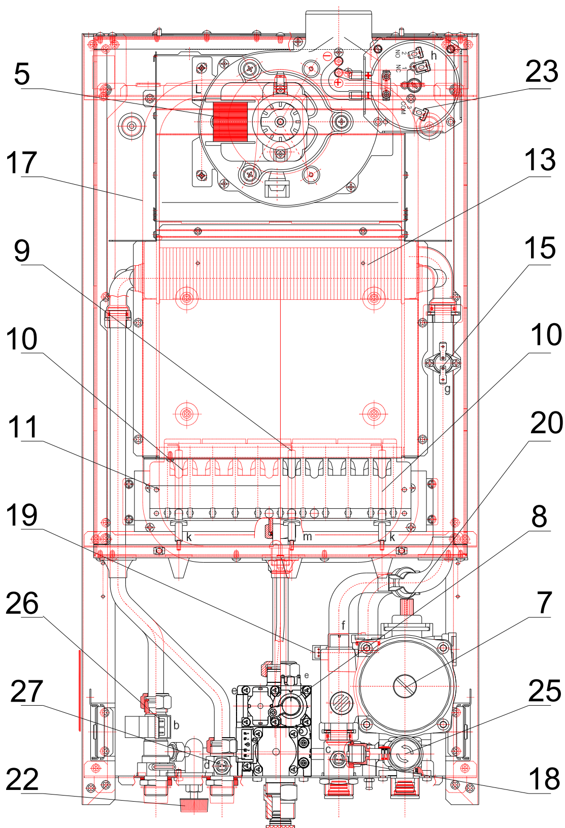
Podstawowe elementy kotła typ Main component of the boiler type Основные элементы котлов типа GCO-DP-21-13
