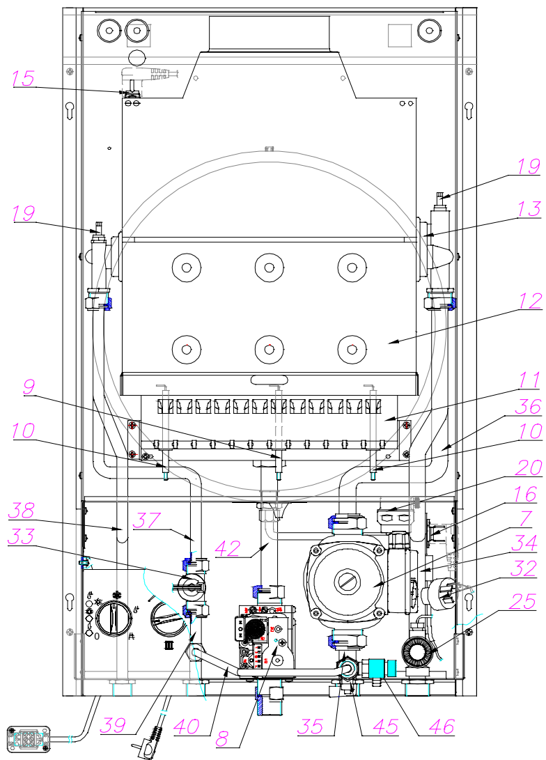
Основные элементы котла типа GCO-DP-23-47
