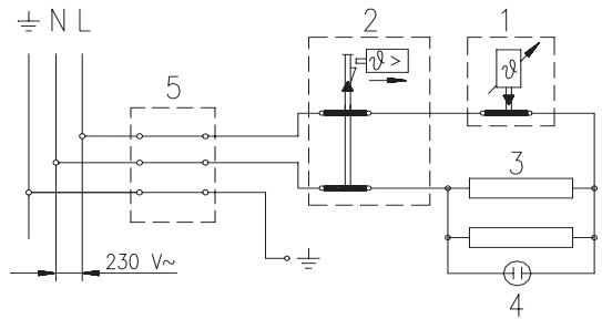
Diagrama eléctrico
