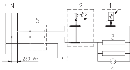
Schéma elektrického zapojenia
