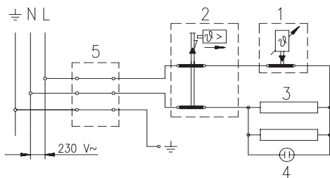
Elektriskā shēma
